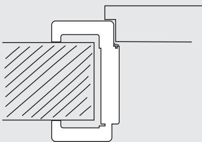
Umfassungszarge
