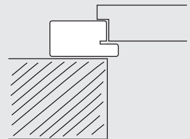
Blendrahmenezarge
